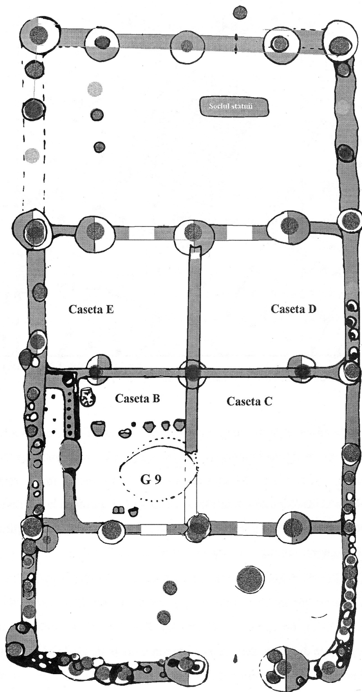
Слика 3: План светилишта бр. 2. Plan of the sanctuary No. 2.
